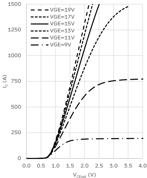
IGBT 输出特性曲线 (典型)
