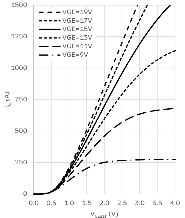
IGBT 输出特性曲线 (典型)
